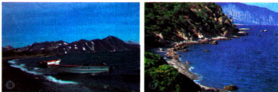
Рис. 132. Побережья Берингова (а) и Черного (б) морей
