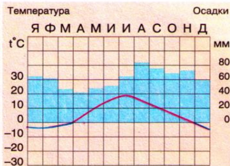
Рис. 125. Умеренный тип климата
