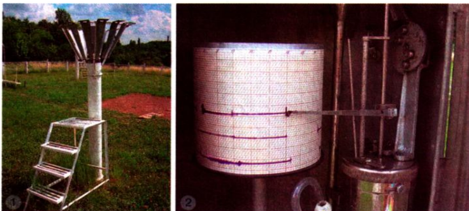
Рис. 110. Осадкомер (1) и плювиограф (2)
