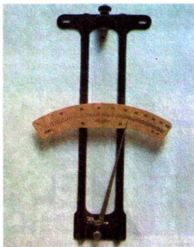
Рис. 104. Волосяной гигрометр
